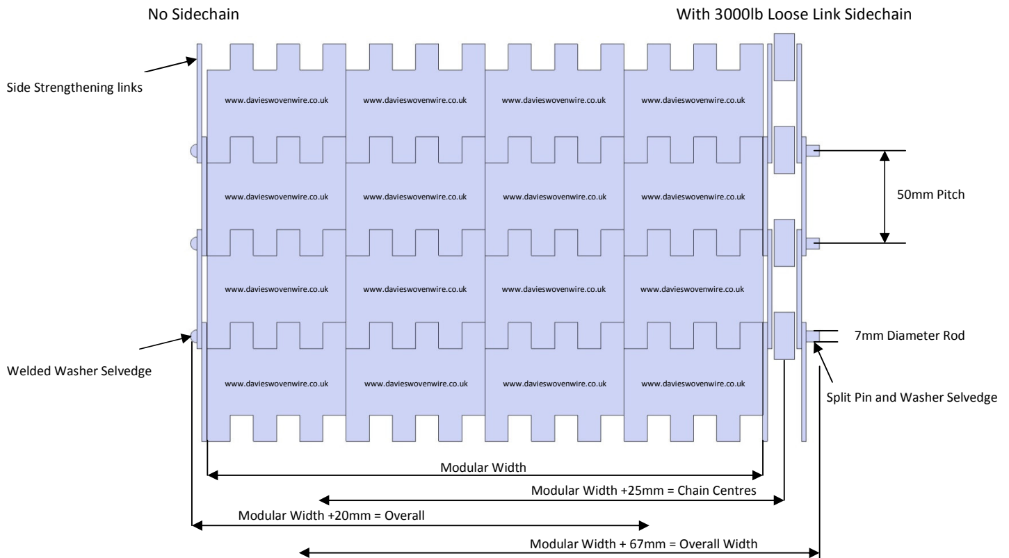
M7 Module
